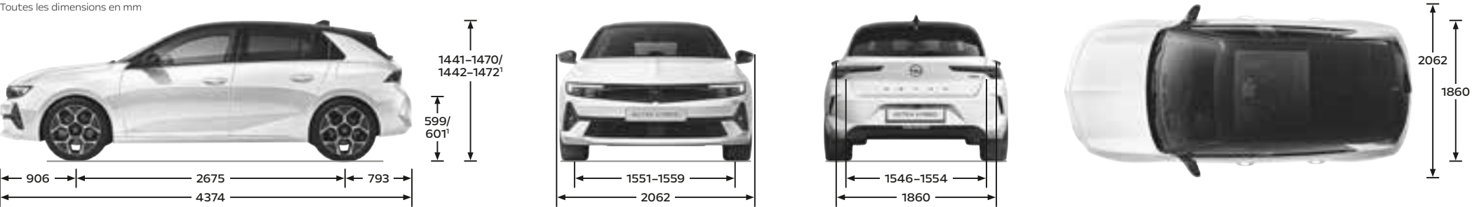
Astra 5 portes Toutes les dimensions en mm
