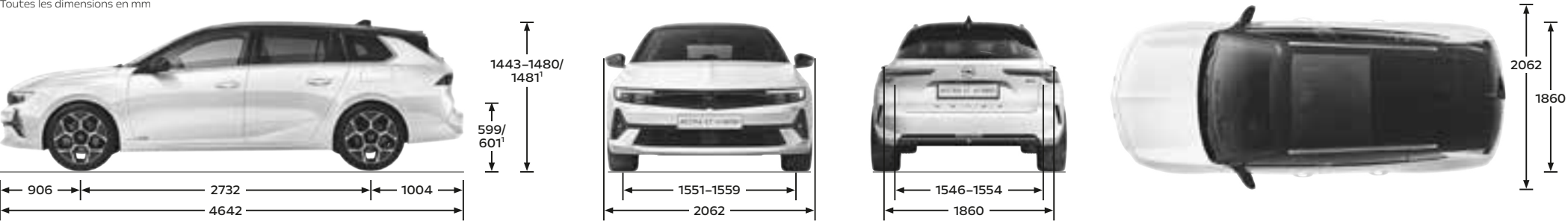
Astra Sports Tourer Toutes les dimensions en mm
