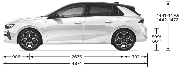
Astra 5-Türer Alle Masse in mm
